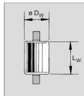
Radialrolle
