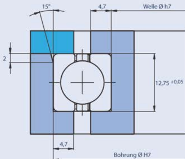
Einbaumaße
