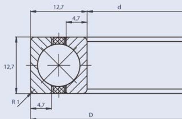
Lagermaße
