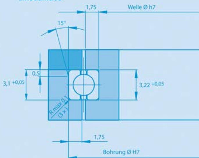
Einbaumaße
